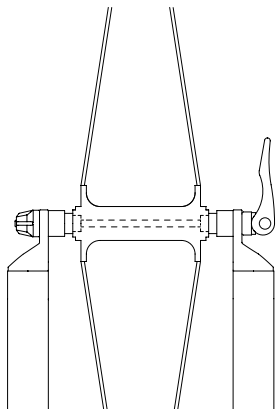
(振れ取り台に前輪ホイールを装着した例)
