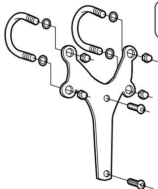
Mounting image (bottle cage is not included) 装着例 (ボトルケージは付属しません)
